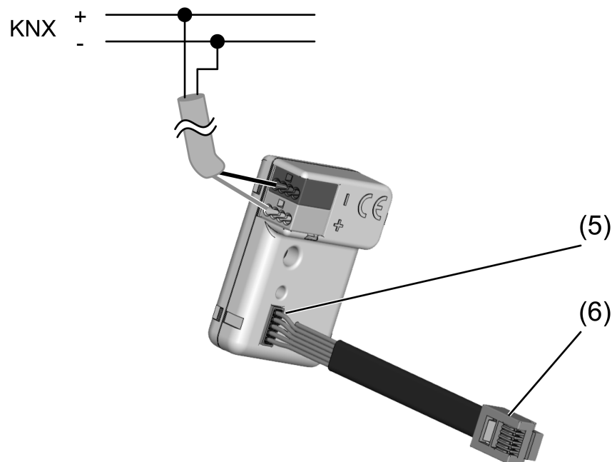
Bild 2: Anschlussbeispiel
