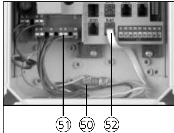
Abb. 7: Anschlüsse in der Steuerung Control 145N
