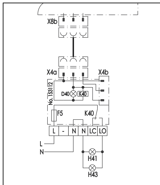
Abb. 22: Schaltplan
