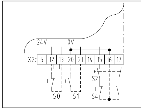
Abb. 16: Schaltplan
