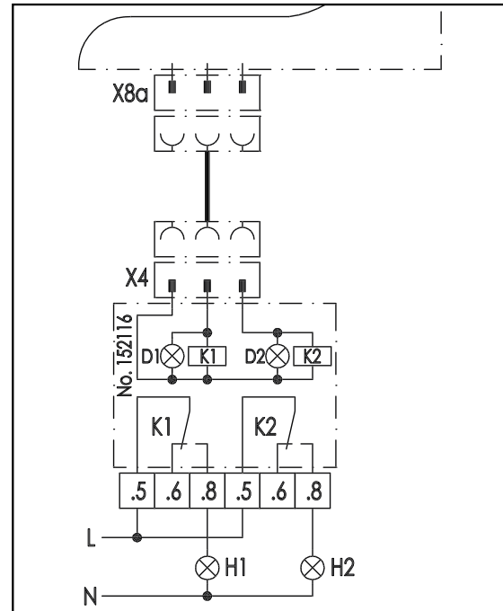
Abb. 21: Schaltplan
