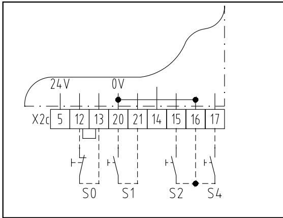
Abb. 15: Schaltplan
