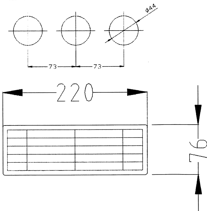
Bohrung für Lüftungsgitter in der Lamelle
